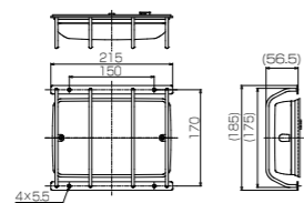
LFA-300専用プロテクター ¥15,000(税別)
