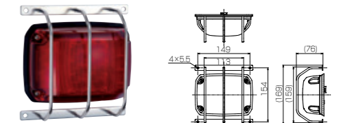
LFA-150専用プロテクター ¥14,000(税別)
