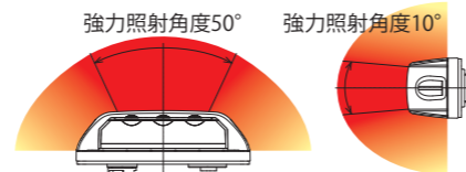
配光図
