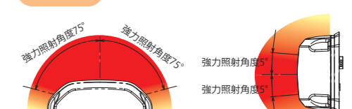
配光図
