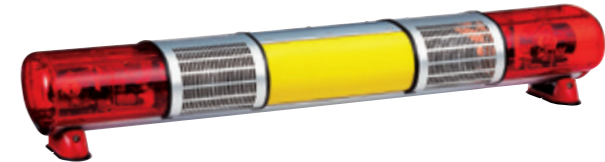
ML 全幅 1305mm 高さ 216mm AD-ML-VA2-H
