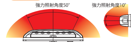
配光図
