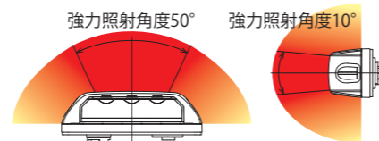
配光図
